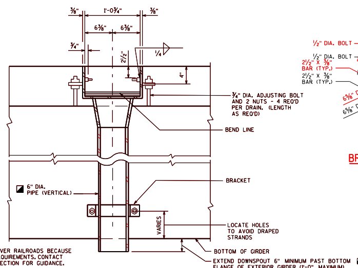
SECTION A2
