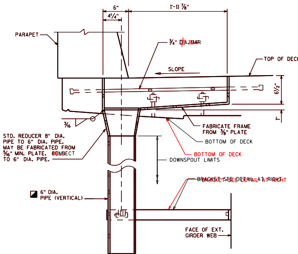
SECTION A1
