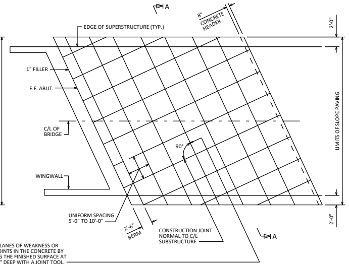
> 15° SKEW
