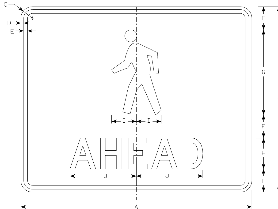
M4-60A
