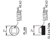
CONDUIT PLUG DETAILS
